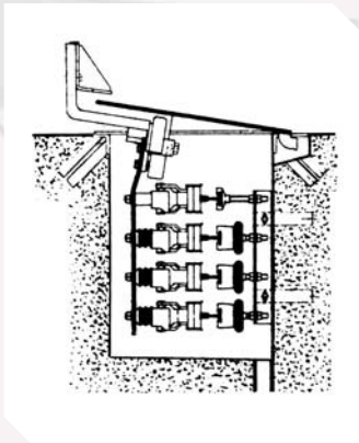
Canal tomacorrientes con carriles conductores de baja tensión
