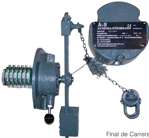
Final de Carrera de contrapeso para control. Counter weight limit switch for control.
