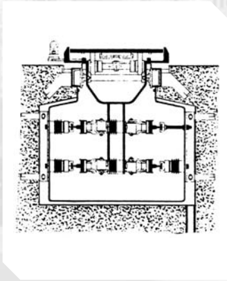
Canal Tomacorrientes con Carriles Conductores. Media Tensión ≤ 6KV.
