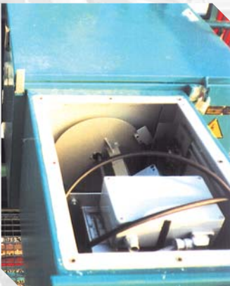
Detalle de colector con 6 fibras ópticas montado en arrollador para cable de 10 KV + 6 fibras ópticas.
