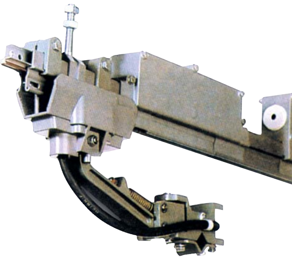
Detalle de carril conductor aislado y pantógrafo tomacorriente.
